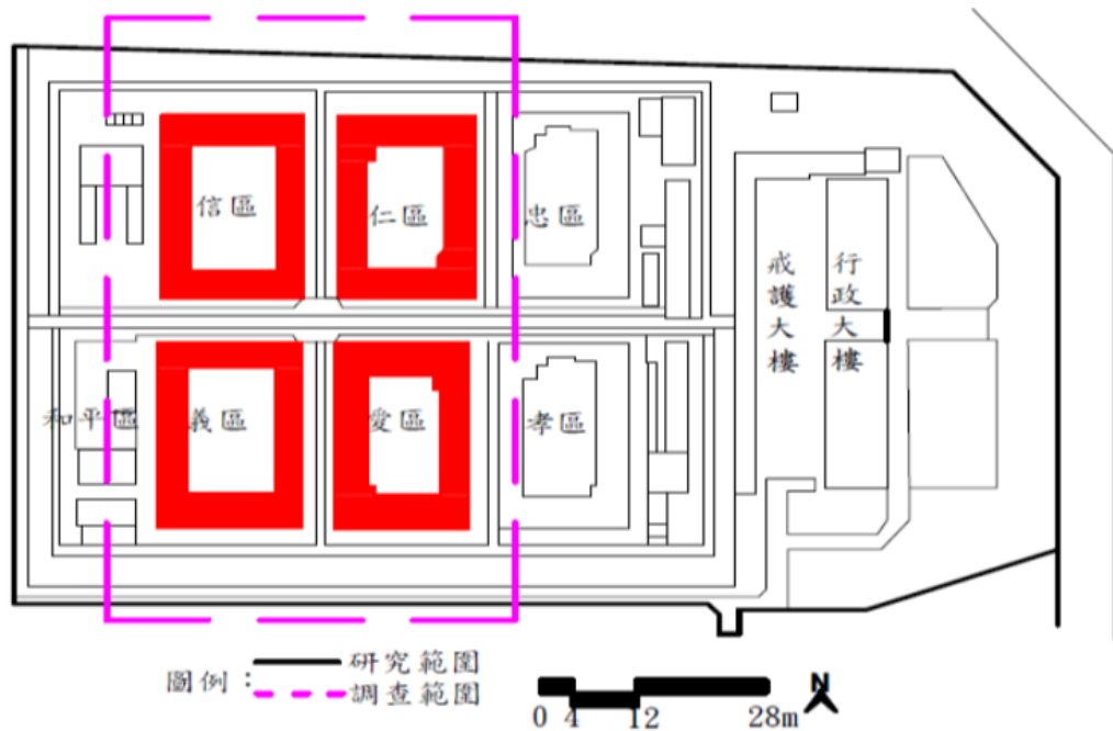
圖 1 臺中監獄整體配置略圖
